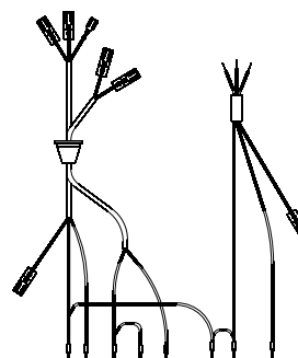
102. Кабель I (комплект) - 3414293 (solo турбо)
